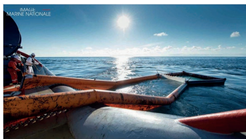
Mise en pêche d'un chalut Thomsea par les marins de la Marine Nationale sur la marée noire du Grande America.
